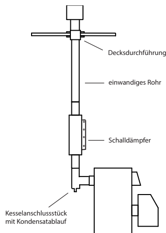
Übersicht eines vertikalen Schornsteins
