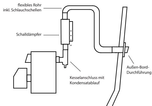
Übersicht eines horizontalen Schornsteins
